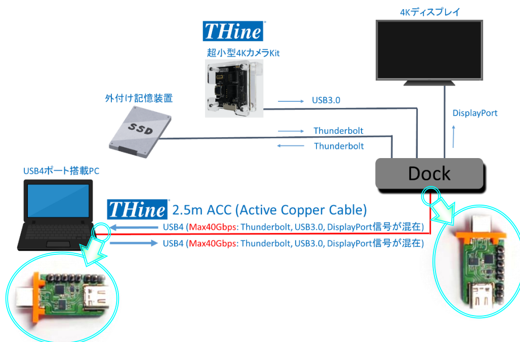
USB4 活用データ伝送距離 3 倍化ソリューションのデモ構成
