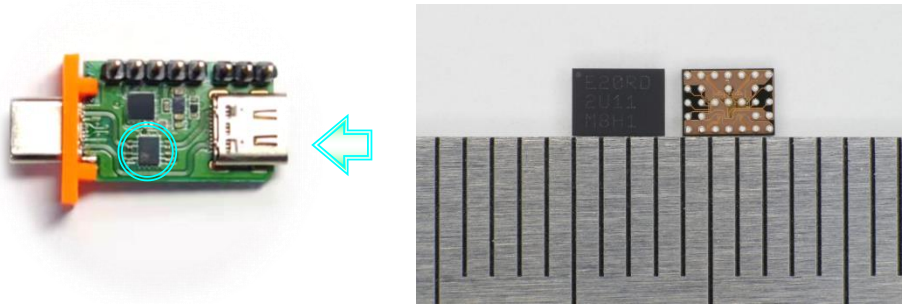
USB4 アクティブケーブル用リドライバ(右写真)搭載エクステンダー(左写真)のサンプル
