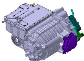
Ni200Ex (200kW/4200Nm)
