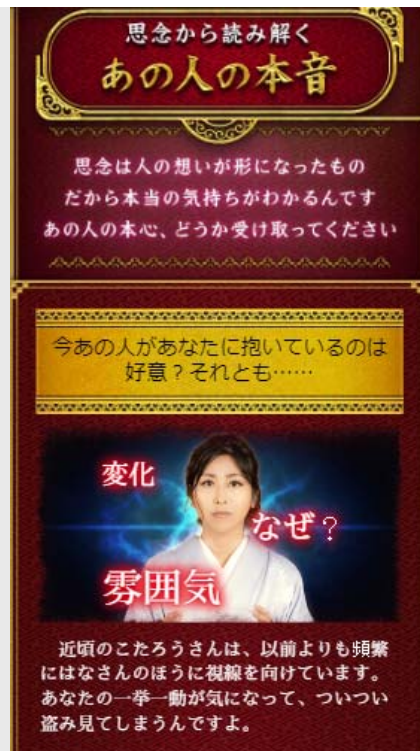
診断結果 3
