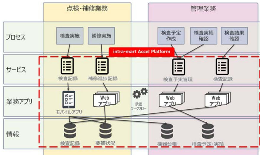
<電気設備保全システムイメージ図>
