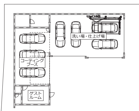
【店舗平面図】
