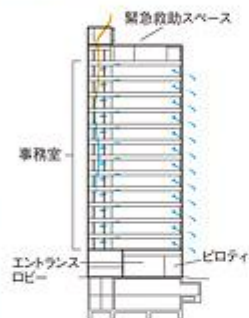
階段室の上下の温度差を利用した自然換気のイメージ図(※)
