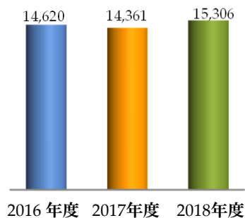
売上高 (1Q)
